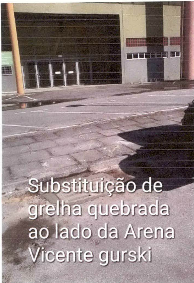
Substituição de grelha quebrada ao lado da Arena Vicente gurski
