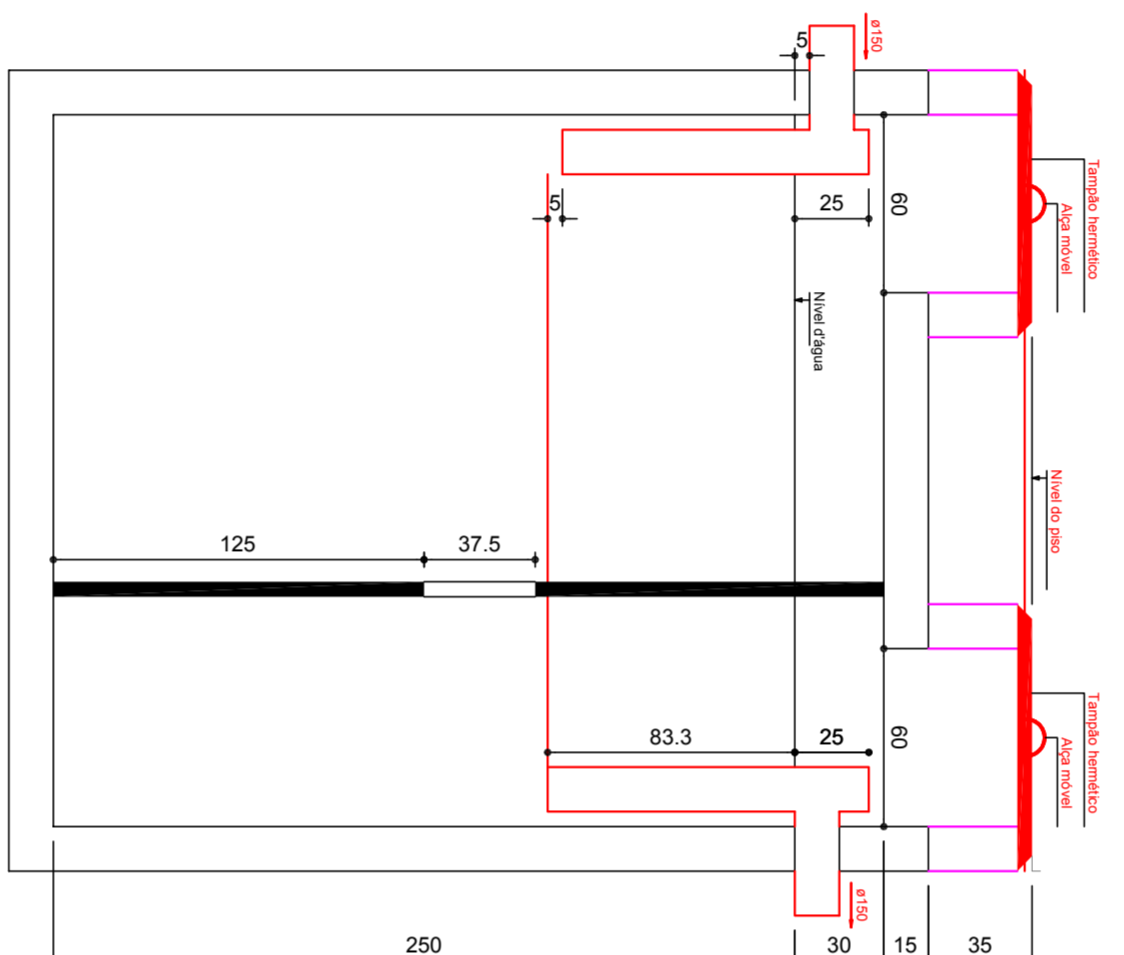
TANQUE SÉPTICO CORTES - ESC. 1:25
