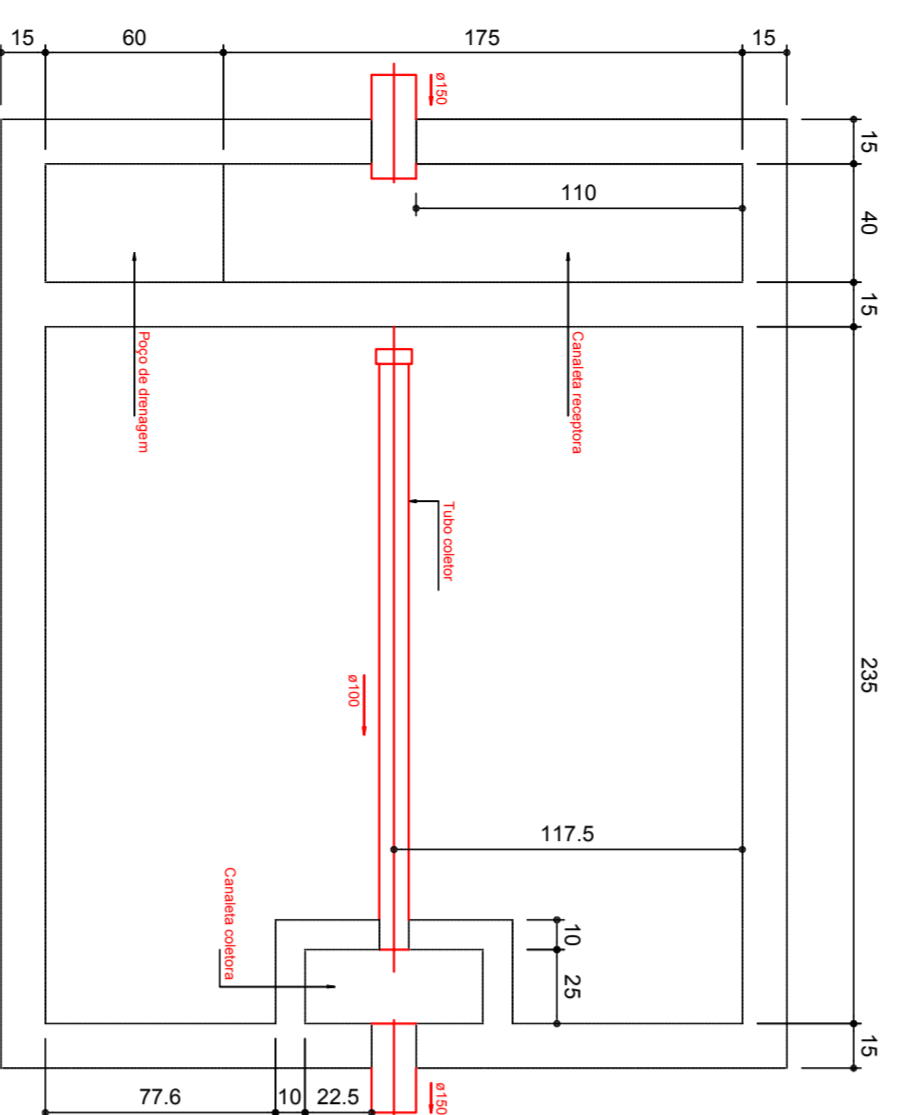
FILTRO ANAERÓBIO PLANTA BAIXA - ESC. 1:25
