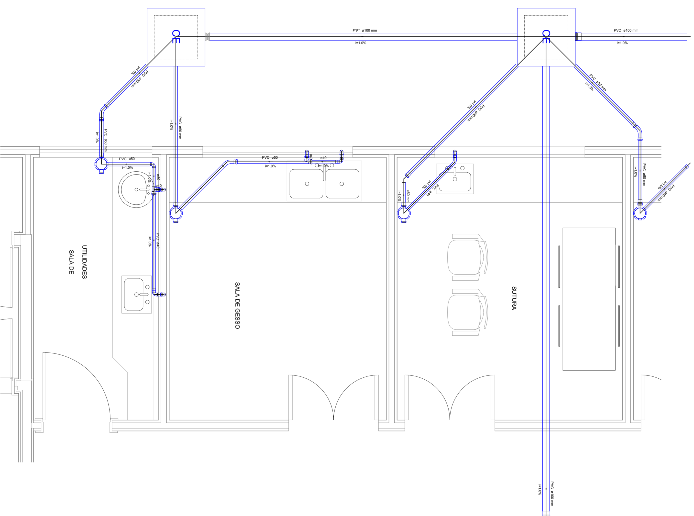
Detalhe S18 escala 1:25
