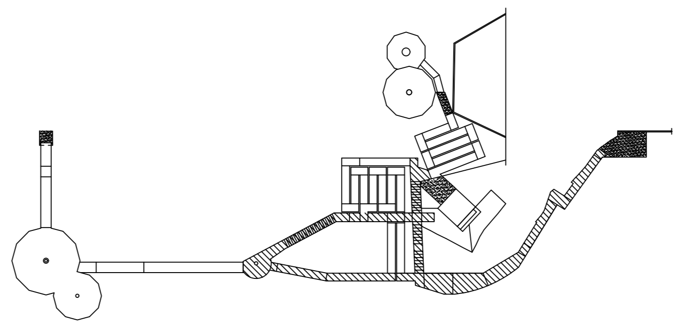
PLANTA DE SITUAÇÃO (TRECHO 2) Esc. 1/100
