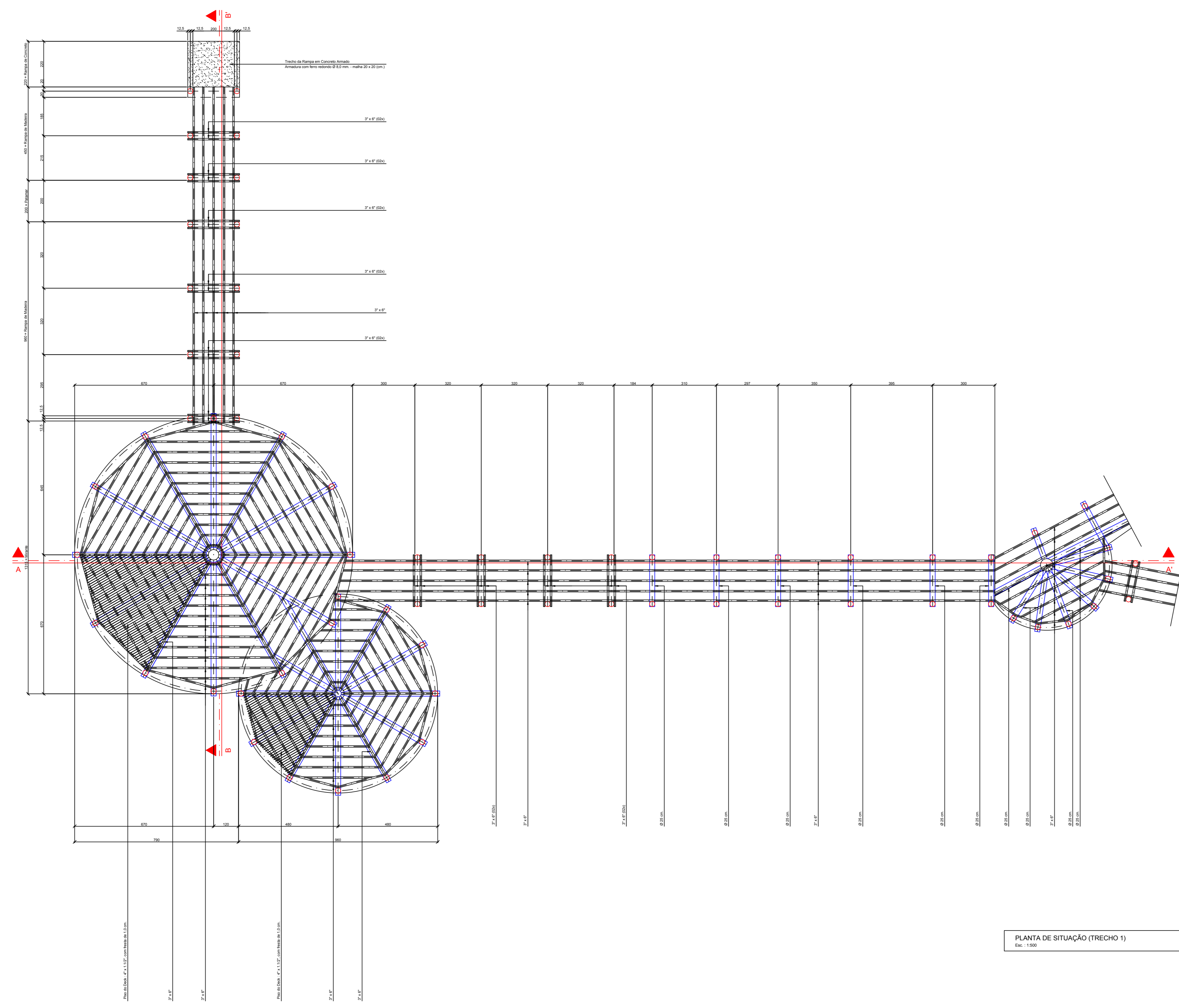
PLANTA BAIXA DA ESTRUTURA DO DECK DA PASSARELA (TRECHO 1) Esc. 1:50
